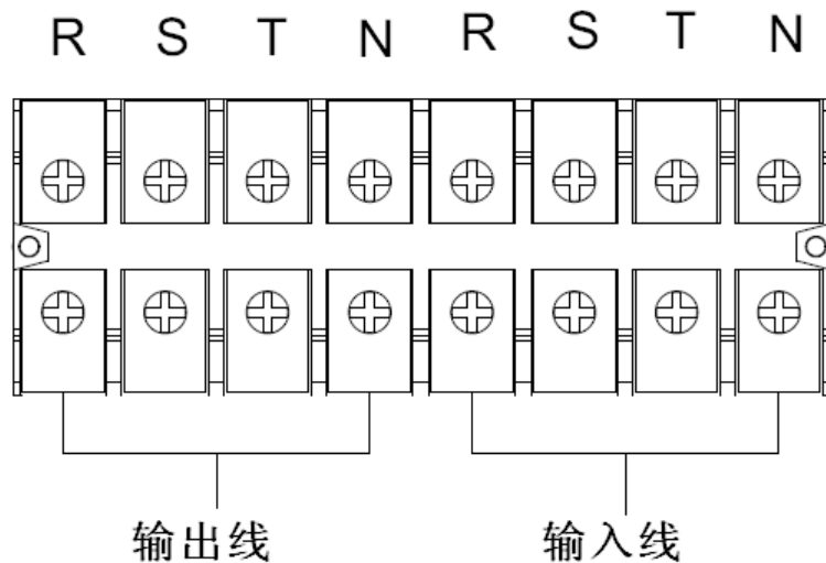
G33-HV 30K(L)/40K(L) and G33-LV 15K(L)/20K(L)端子排示意图
