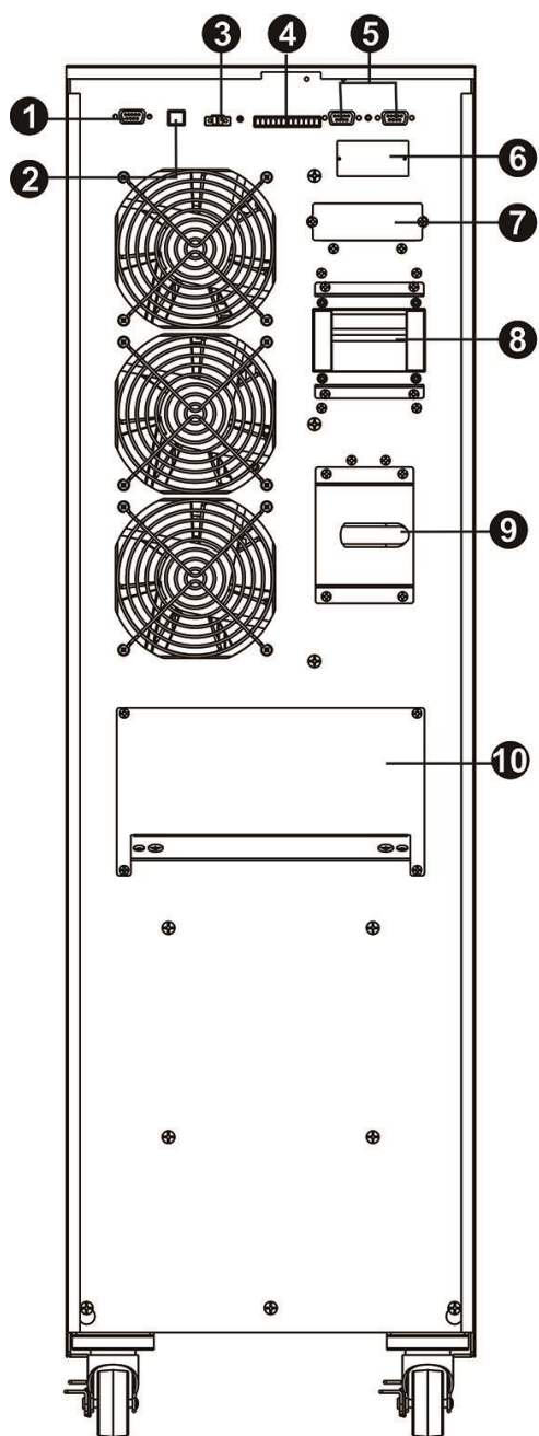
图1: G33-HV 30K(L)/G33-LV 15K(L)背板
