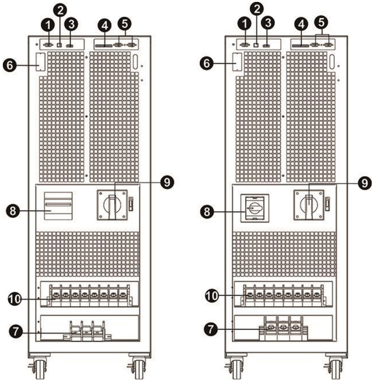
图4: G33-HV 60KL/LV 30KL 打开来前面板视图 图5:G33- HV 80KL/LV 40KL 打开来前面板视图
