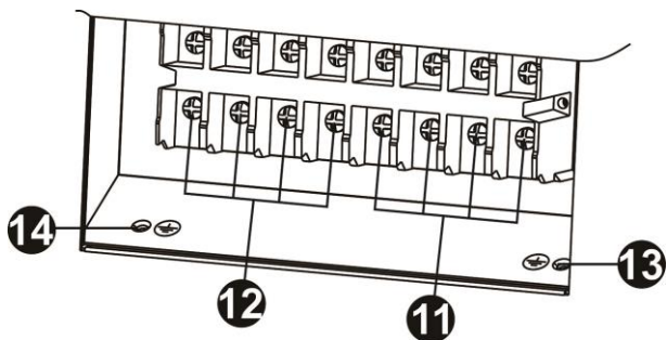
图3: G33-HV 30K(L)/LV 15K(L)/ HV 40K(L)/LV 20K(L) 输入/输出端子
