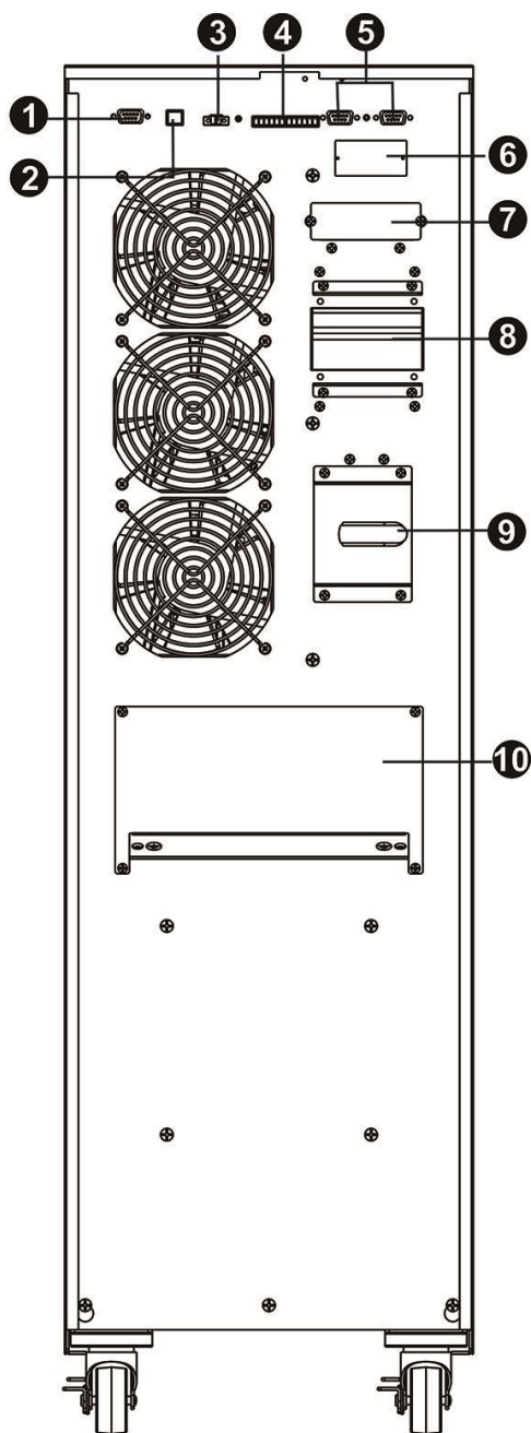
图2: G33-HV 40K(L)/G33-LV 20K(L)背板
